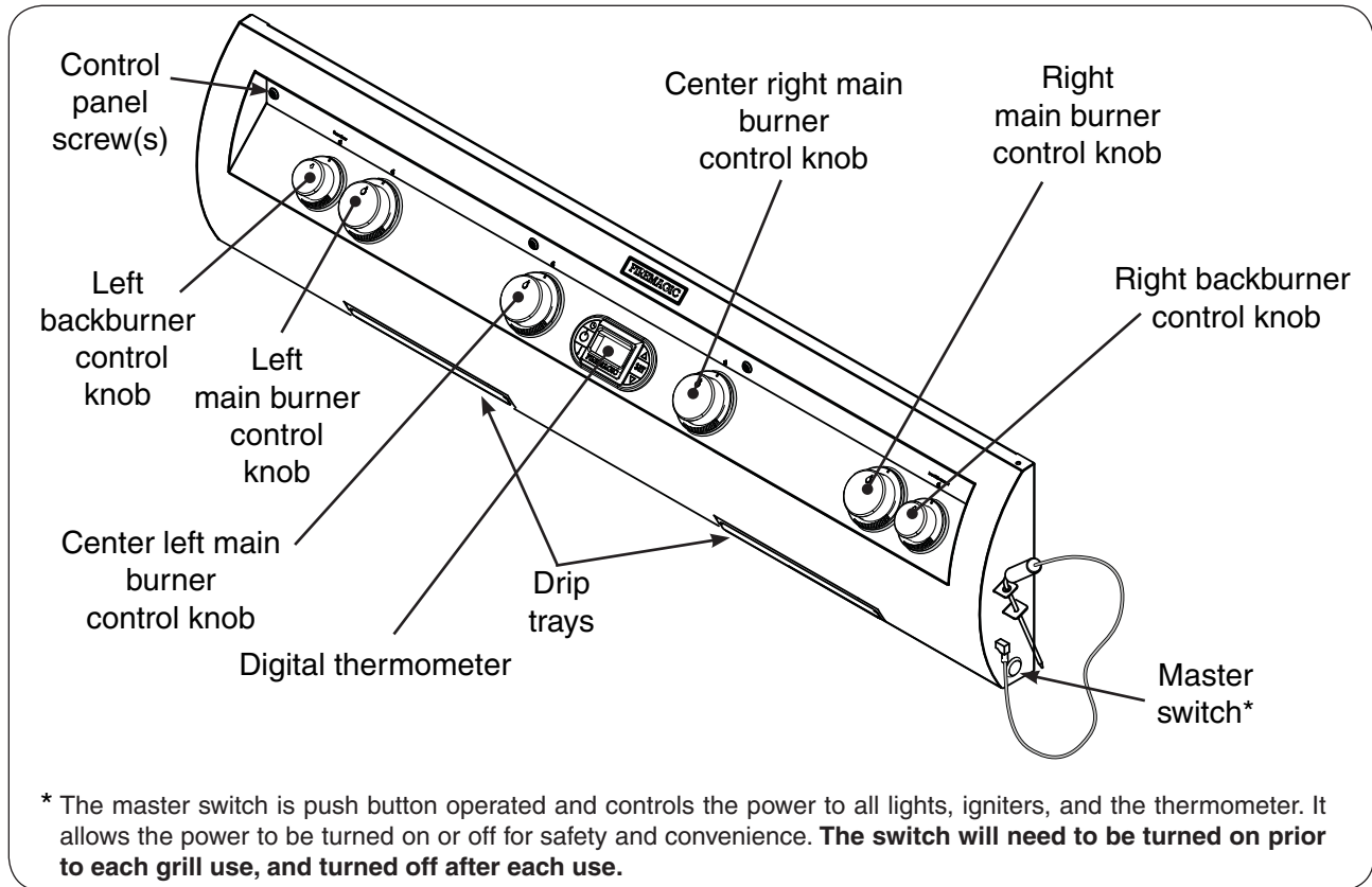
Fig. 22-1 E1060i controls
